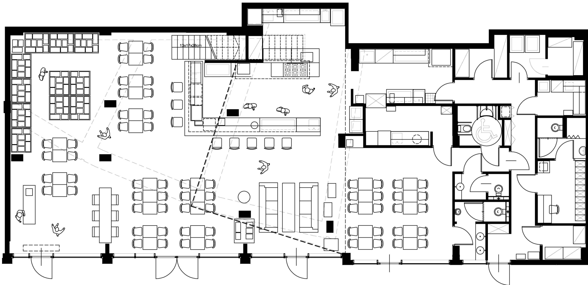
RZUT PARTERU
